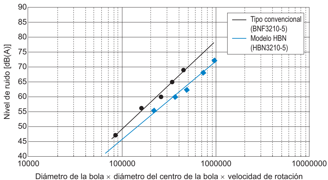
Fig.2 Nivel de ruido del husillo de bolas
