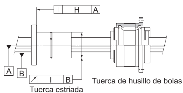
Tuerca estriada
