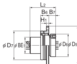
Eje nervado (Modelos BNS 1616A a 4040A)
