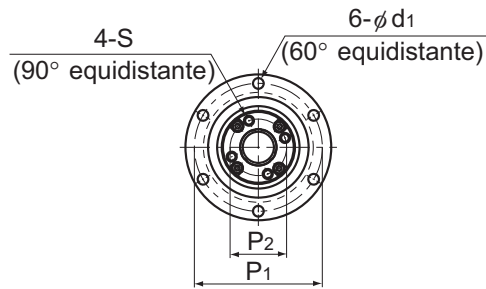
Husillo de bolas (Modelos BNS 1616A a 4040A)
