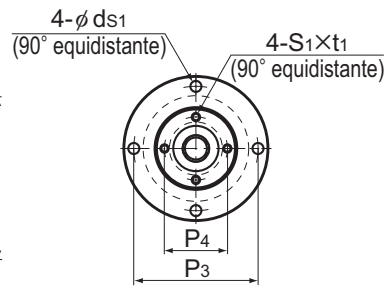
Eje nervado (Modelos BNS 0812A y 1015A)
