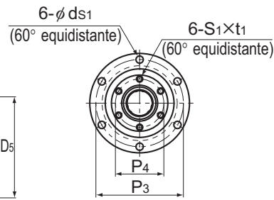
Eje nervado (Modelos BNS 1616A a 4040A)
