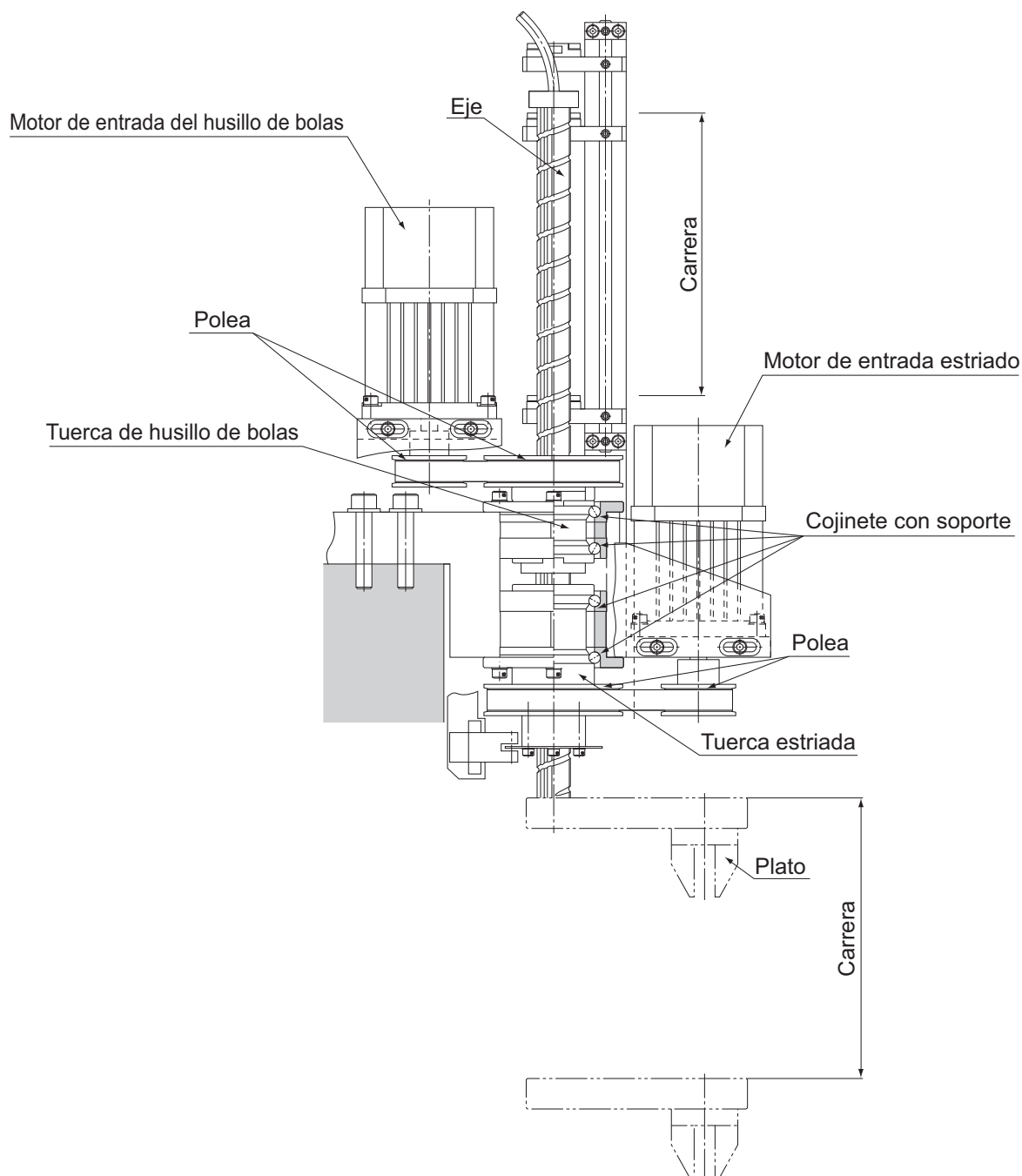
Fig.5 Ejemplo de uso de modelo BNS
