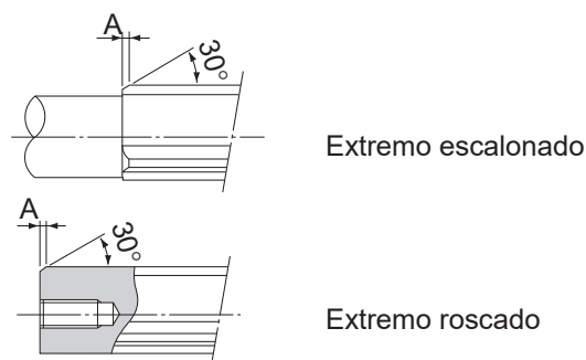
Fig.2 Inglete A
