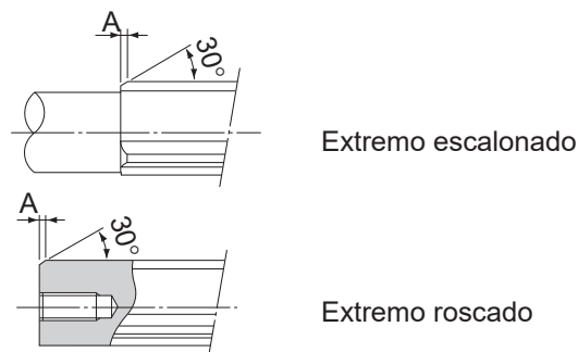
Fig.2 Inglete A
