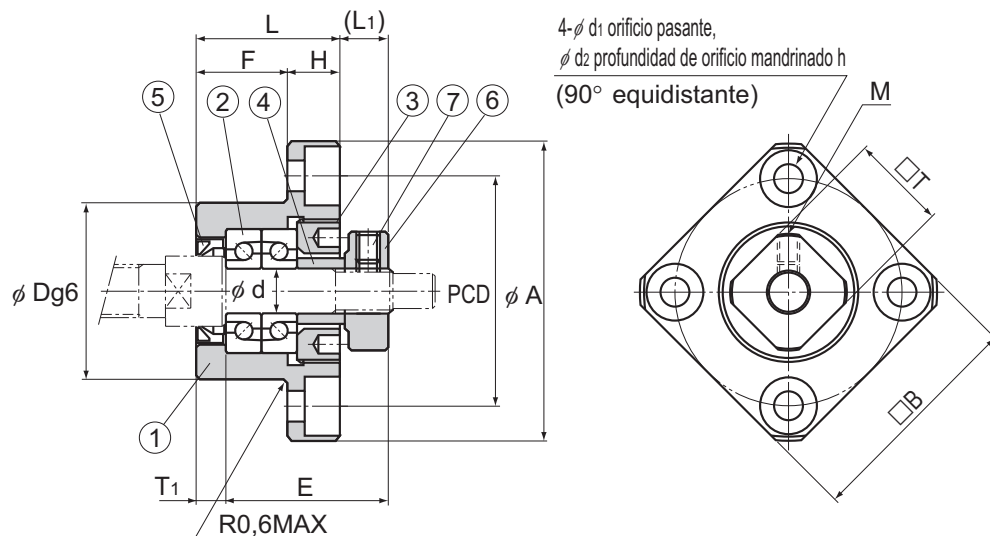
Método de montaje A
