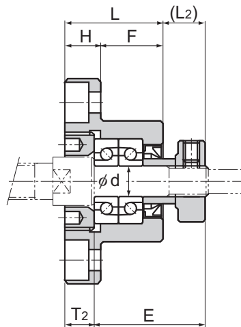
Método de montaje B
