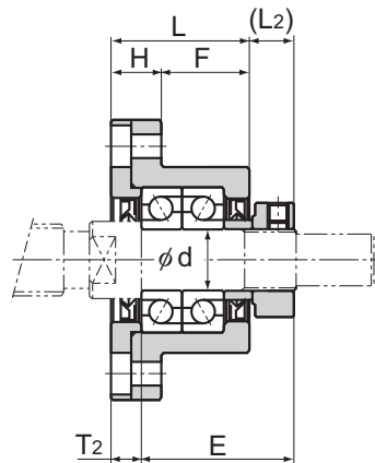
Método de montaje B
